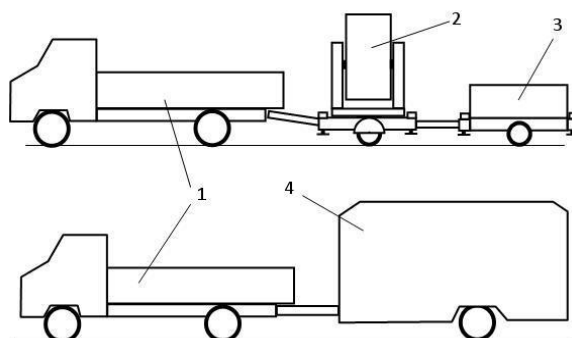
Рис. 1. Буксируемый вариант МПВ в походном положении
