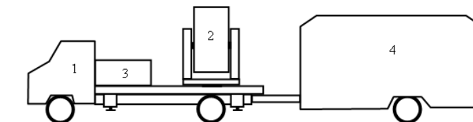
Рис. 2. Самоходный вариант МПВ № 1 с буксируемым жилым модулем в походном положении
