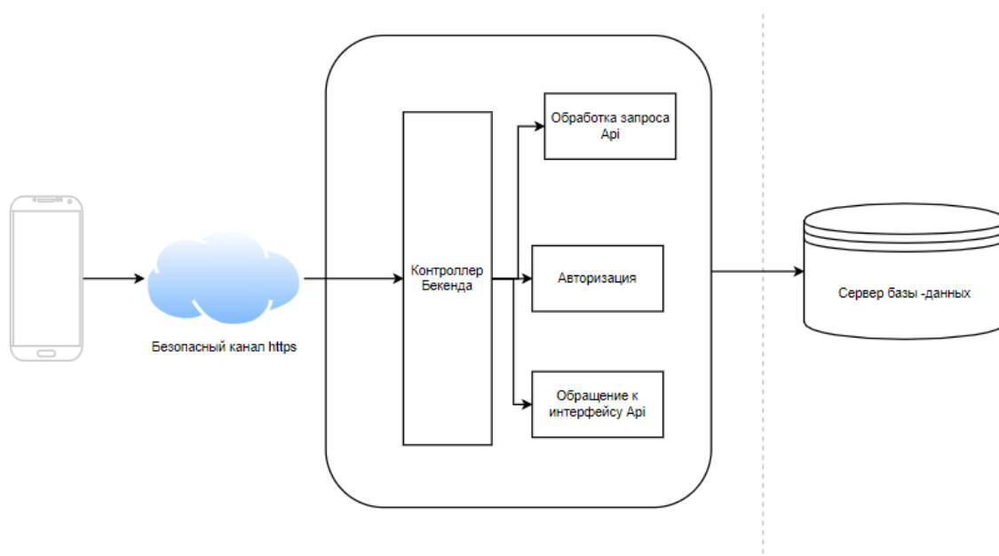
Рисунок 1 –Архитектура бекенда
