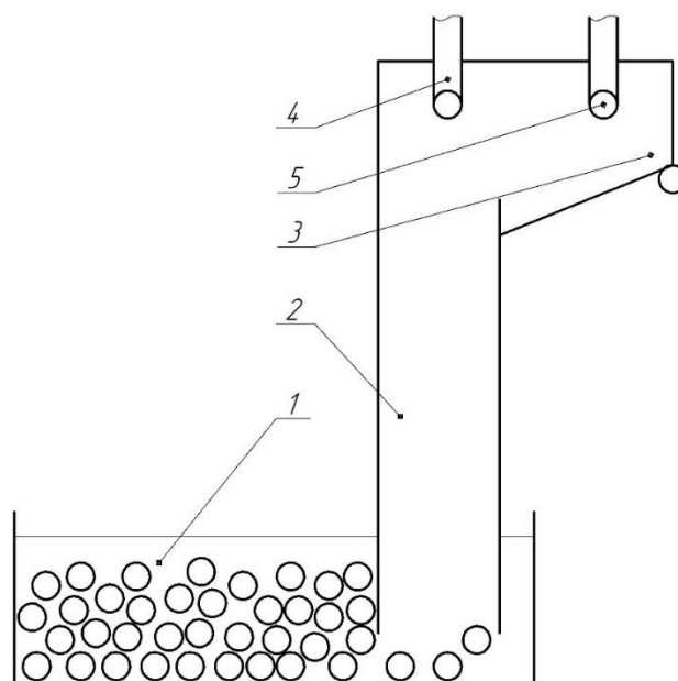
Рис.1 – Схема пневматического высевающего аппарата точного высева без подвижных частей
