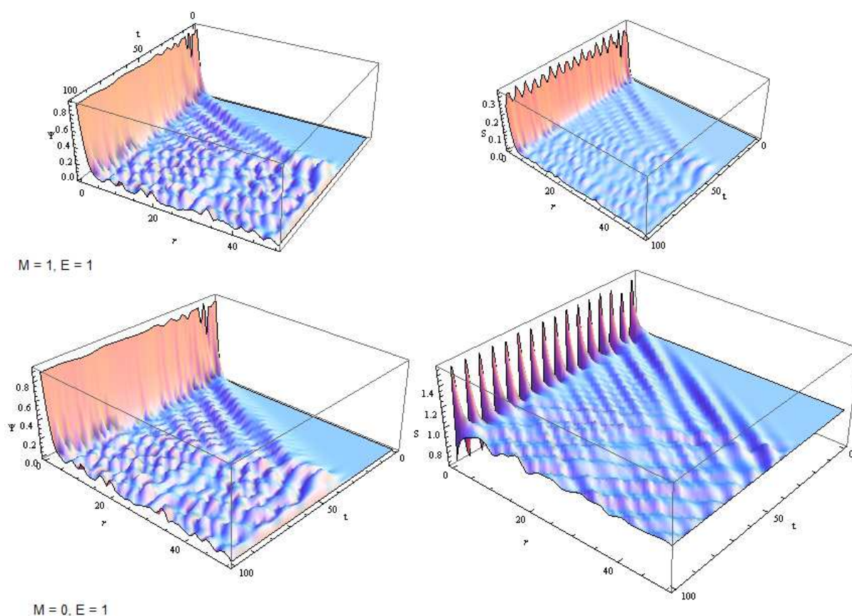
Рис. 4. Моделирование гравитационных волн на основе модели (45) и действия системы по уравнению (32) при большом значении параметра B = 1 .
