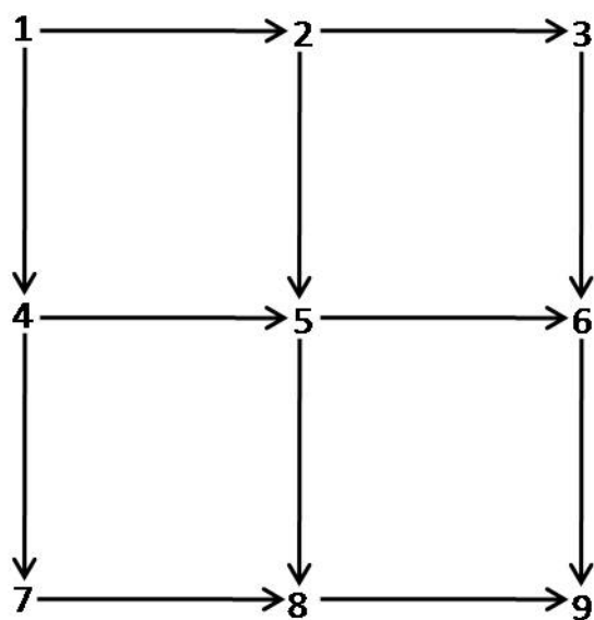
Рисунок 1 Иерархическая структура группы птицы, состоящей из 9 особей
