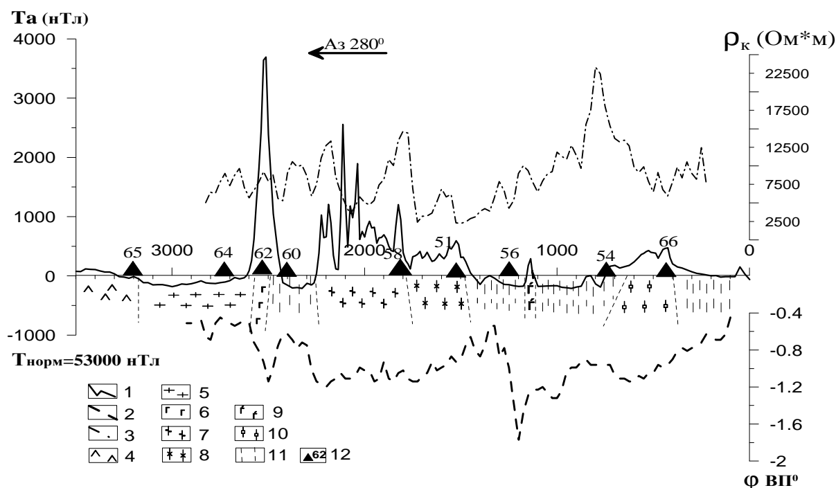
Рис. 2. Результаты геофизических наблюдений по профилю Каппала-Горное.
