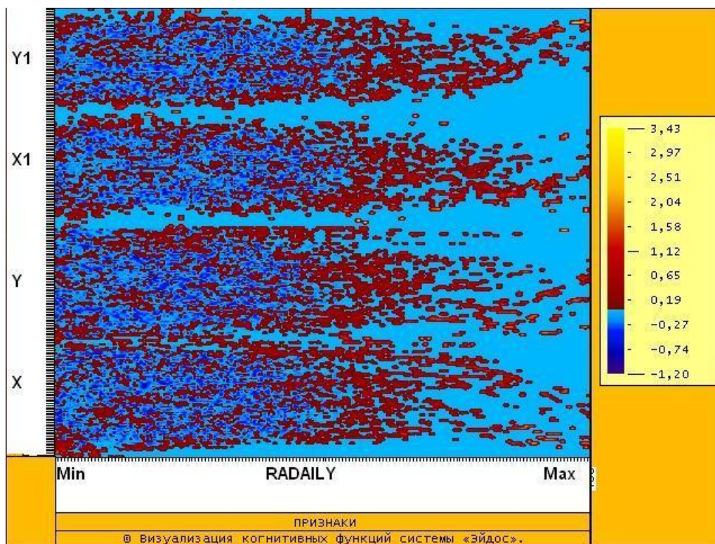
Рис. 8. Зависимость координат и угловой скорости движения полюса Земли от параметра RADAILY
