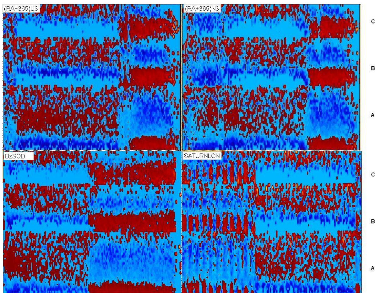
Рис. 3. Зависимость частоты категорий однократных (А), двукратных (В) и трехкратных (С) сейсмических событий с магнитудой m_b \geq 4 от параметра P3 вычисленного для Урана и Нептуна при Q_{0i} = 365 , долготы Сатурна и вариаций вертикальной компоненты индукции магнитного поля Земли на станции SOD в 1963-2006 гг по данным /10/ в модели M160.
