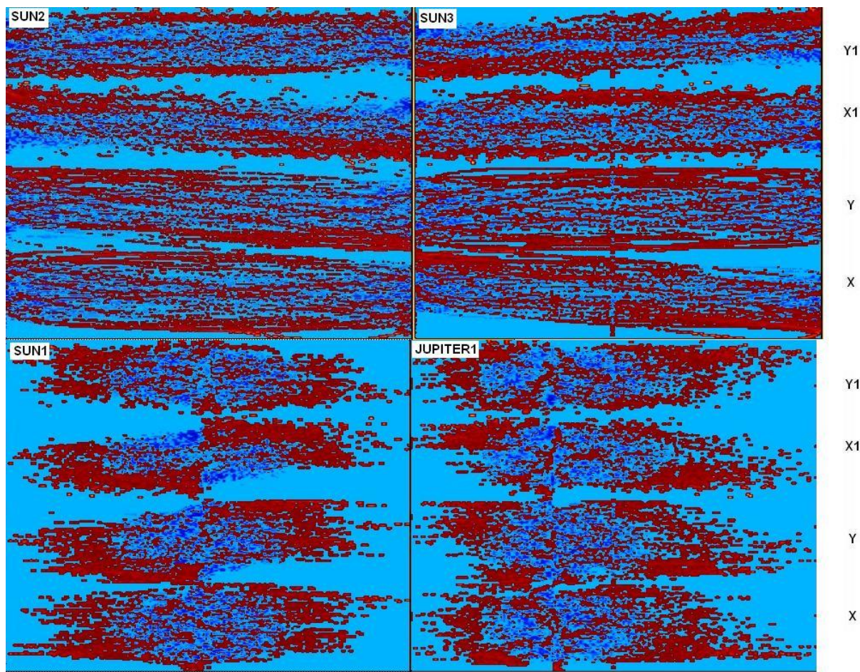
Рис. 10. Зависимость координат и угловой скорости движения полюса Земли от параметров SUN2, SUN3, вычисленных по уравнениям (9) при Q=1 и от параметров SUN1, JUPITER1, вычисленных при Q_0=0 .
