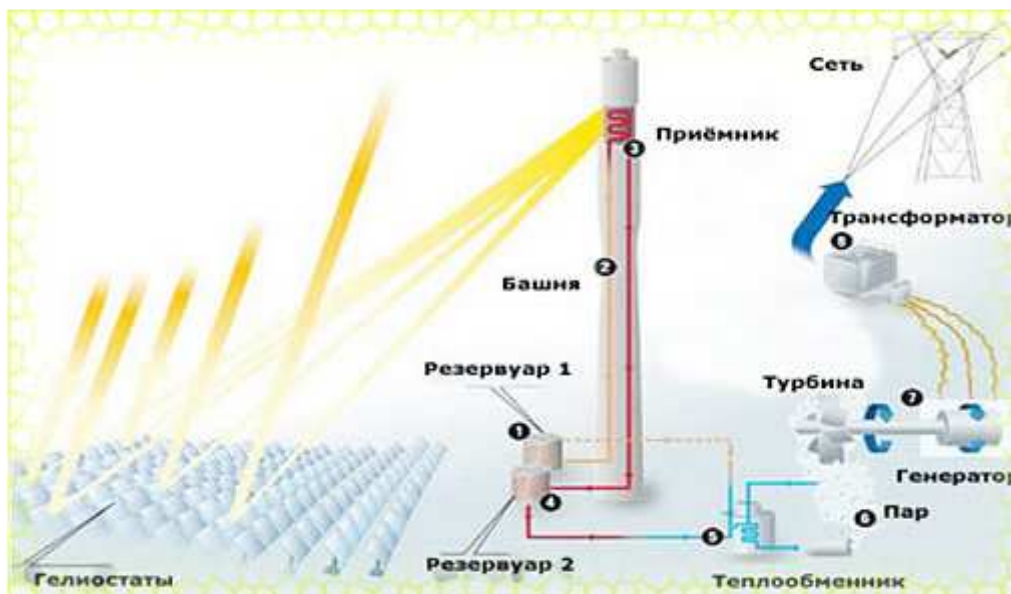
Рисунок 5 – Солнечный коллектор башенного типа
