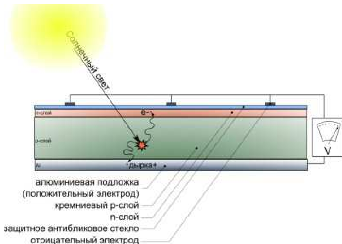
Рисунок 3 – Устройство фотоэлектрического элемента
