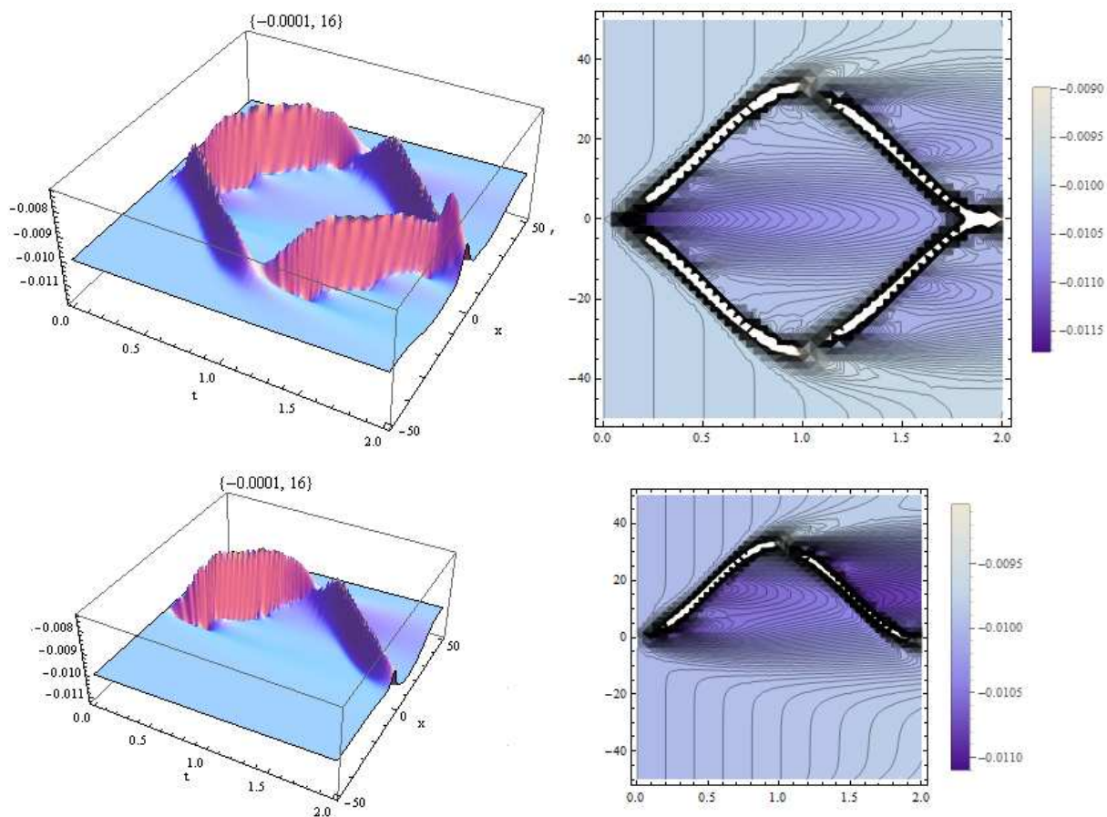
Рис. 6. Отображение движения тел в метрике (6) на основе одномерной модели (17): a = 16; \omega = \pi; q_0 = 10^{-4}, U_0 = -10^{-2} .
