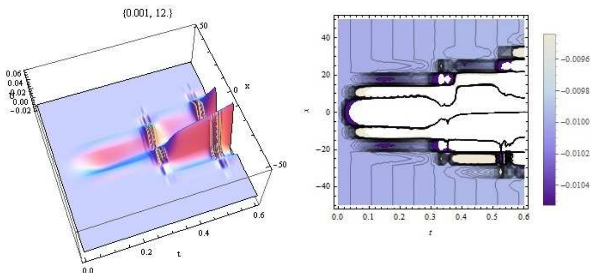
Рис. 7. Развитие неустойчивости в модели (17) при движении двух тел в метрике (6). Расчеты выполнены на основе четырехмерной модели (17): a = 12; \omega = \pi; q_0 = 10^{-3}, U_0 = -10^{-2} .
