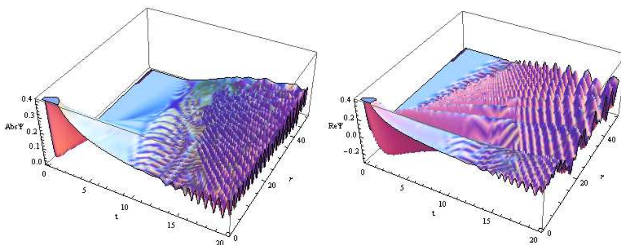
Рис. 3. Распад начального состояния в модели (29).
