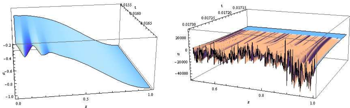
Рис. 1. Переход к геометрической турбулентности в модели (35).
