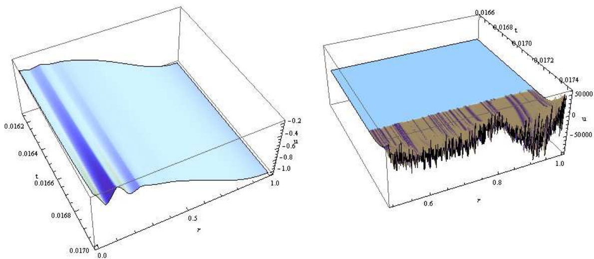
Рис. 2. Переход к геометрической турбулентности в модели (38).
