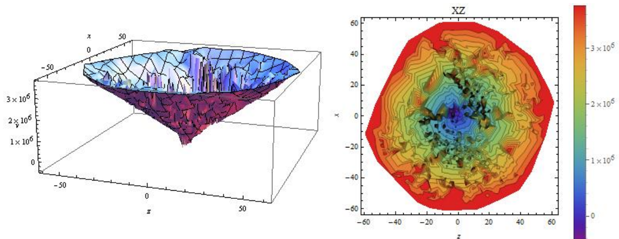
Рис. 5. Изолинии радиальной компоненты скорости (м/с) в зависимости от расстояния в мегапарсеках в проекции на плоскость XZ в масштабе 125 мегапарсек.
