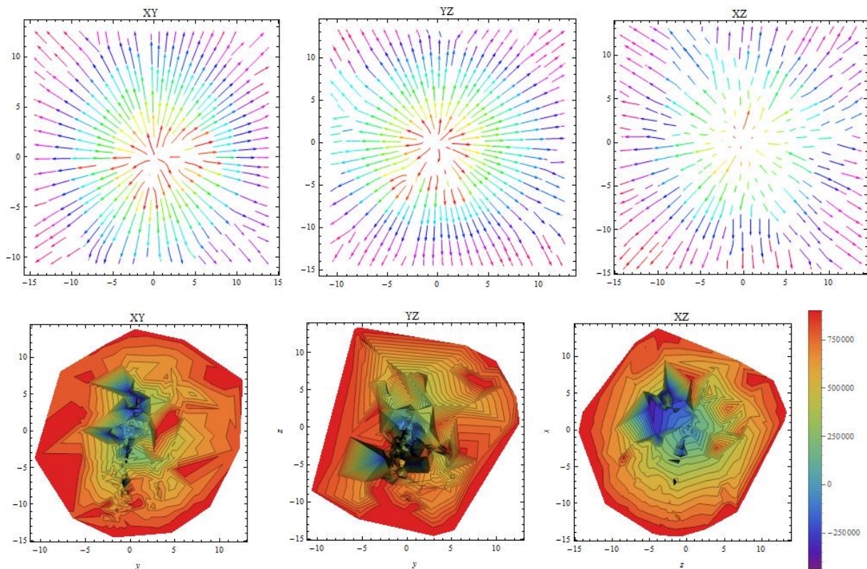
Рис. 4. Течение в ближней зоне в масштабе 25 мегапарсек: хорошо видны зоны возвратного течения, в котором красное смещается на синее, то есть скорость течения меняет знак. На нижних рисунках показаны изолинии радиальной компоненты скорости (м/с) в зависимости от расстояния в мегапарсеках.
