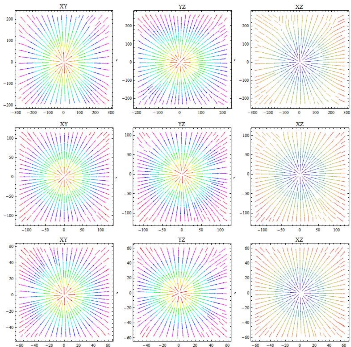
Рис. 3. Проекция течения (16) на плоскости куба в масштабе 500, 250 и 125 мегапарсек: во всех масштабах хорошо просматривается радиальное течение (16).
