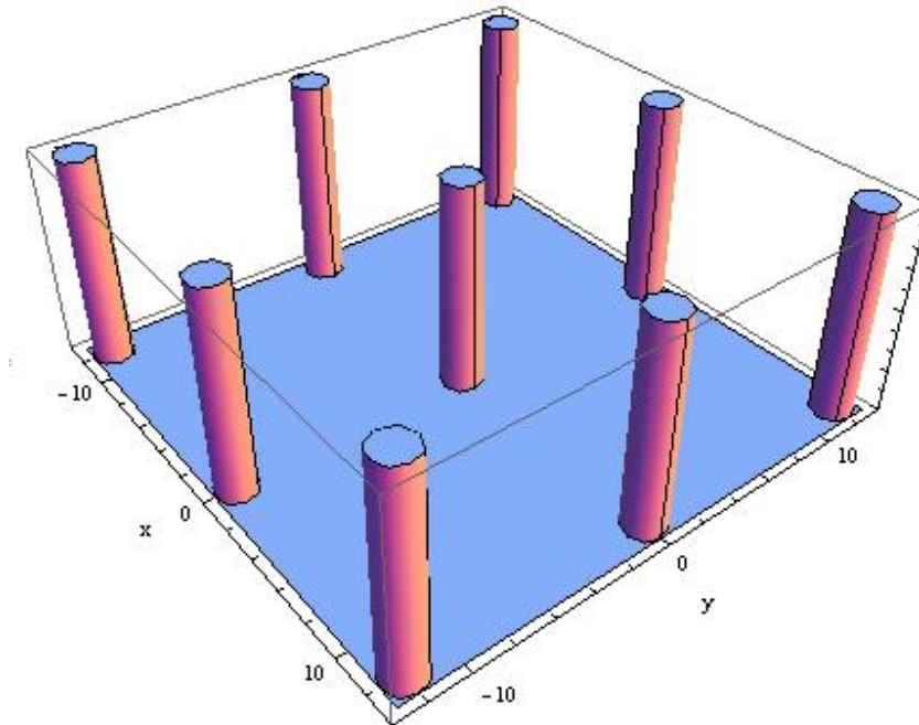
Рис. 2. Система труб, образующих решетку с шагом L = 12 .
