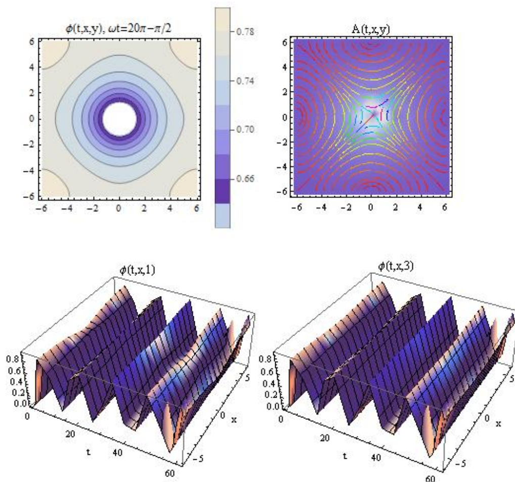
Рис. 4. Формирование волнового поля скалярного и векторного потенциалов в системе с L/R=100 . Характерное волновое число k = w/c = 1/12 ; g = 0.01 . На нижних рисунках показана развертка потенциала в двух сечениях: y = 1; 3 .
