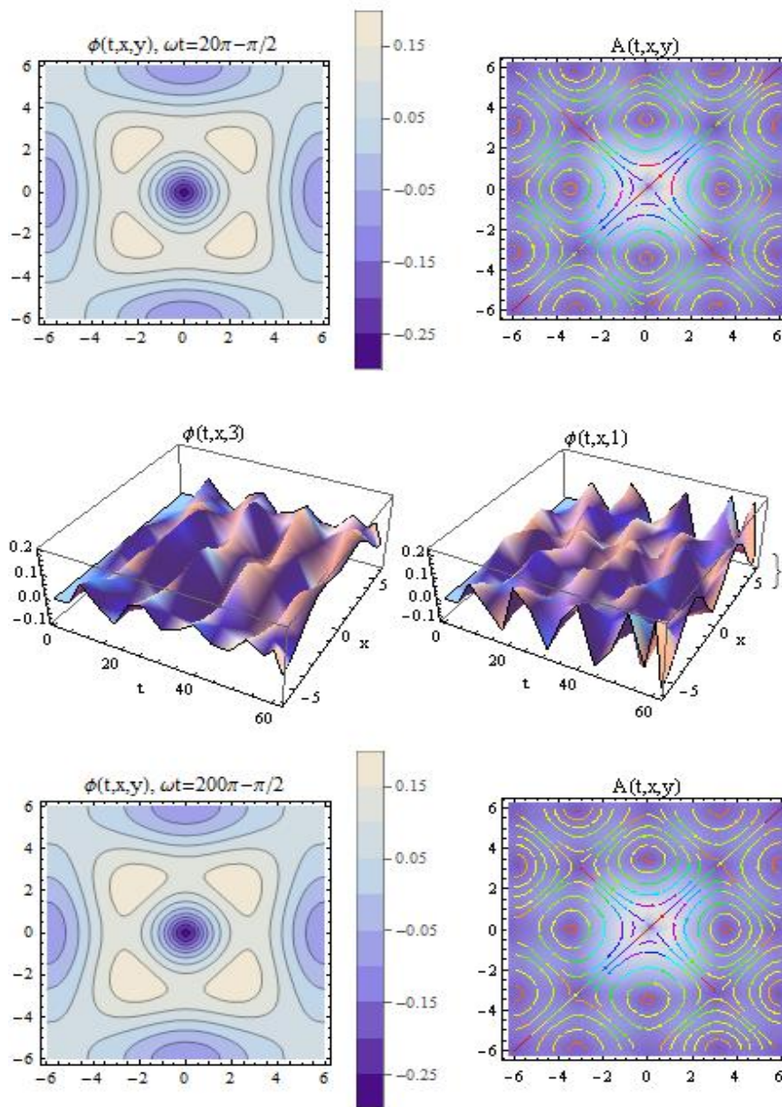
Рис. 5. Стабилизация волнового поля в системе с параметрами L/R = 100 , k = w/c = 1 ; g = 0.1 . На средних рисунках показана развертка потенциала в двух сечениях: y = 1; 3 .
