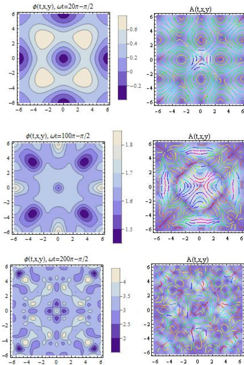
Рис. 3. Формирование волнового поля скалярного и векторного потенциалов в системе с шагом решетки L = 12 , радиусом трубы R = 0.06 и с характерным волновым числом k = w/c = 1 ; g = 0 .
