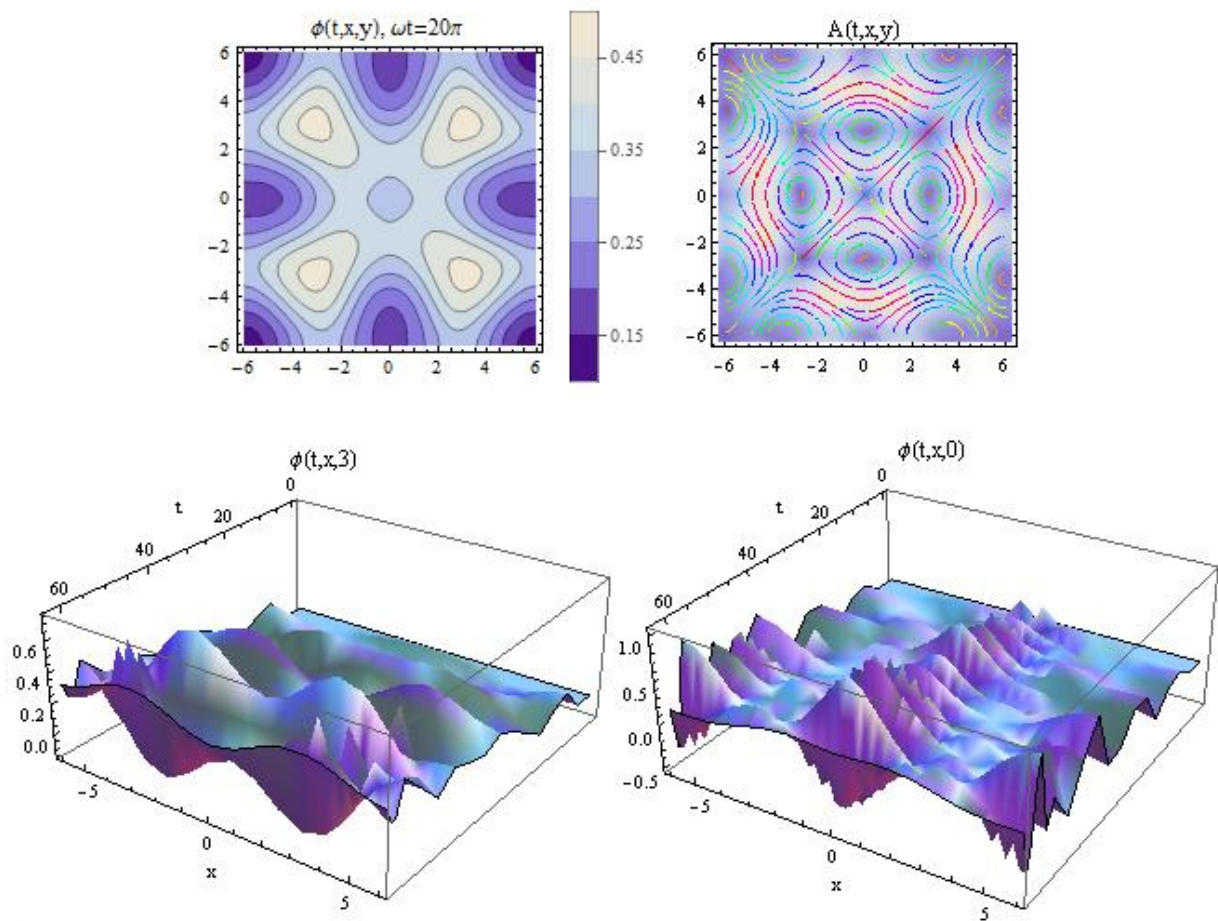
Рис. 6. Формирование волнового поля скалярного и векторного потенциалов в системе с шагом решетки L = 12 и радиусом трубы R = 0.06 : амплитуда потенциала в сечении трубы достигает значения 1 за 10 периодов колебаний (нижний правый рисунок). Волновое число k = w / c = 1 ; g = 0 .
