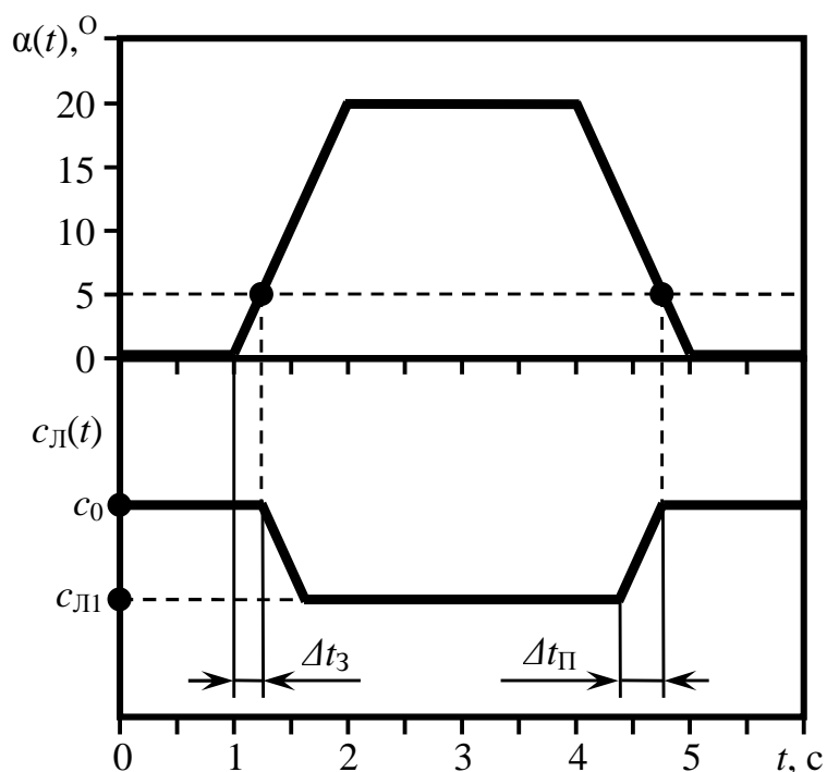
Рисунок 3. Графики управления в процессе компьютерного эксперимента углом поворота колес автопоезда \alpha(t) и жесткостью пневматической подвески по левому борту c_L(t)
